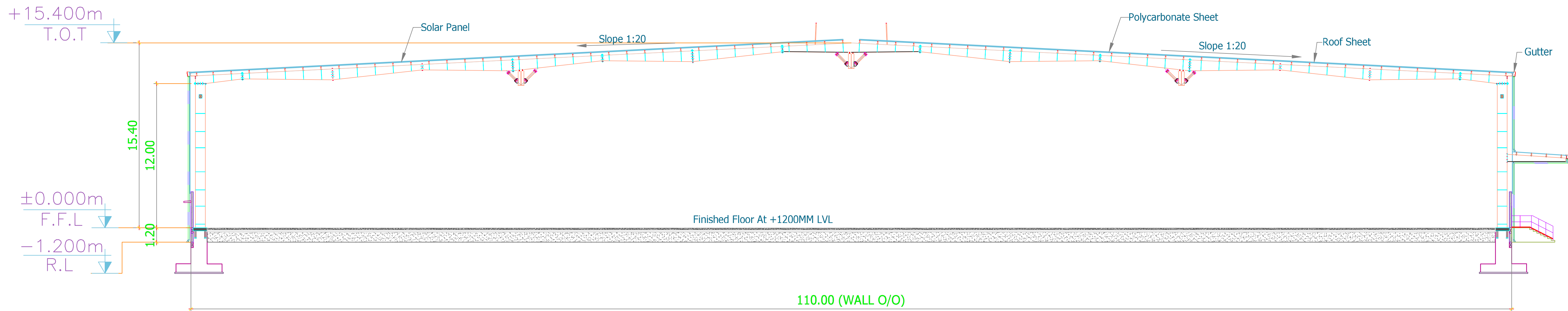
Section "B-B" BLOCK A3
