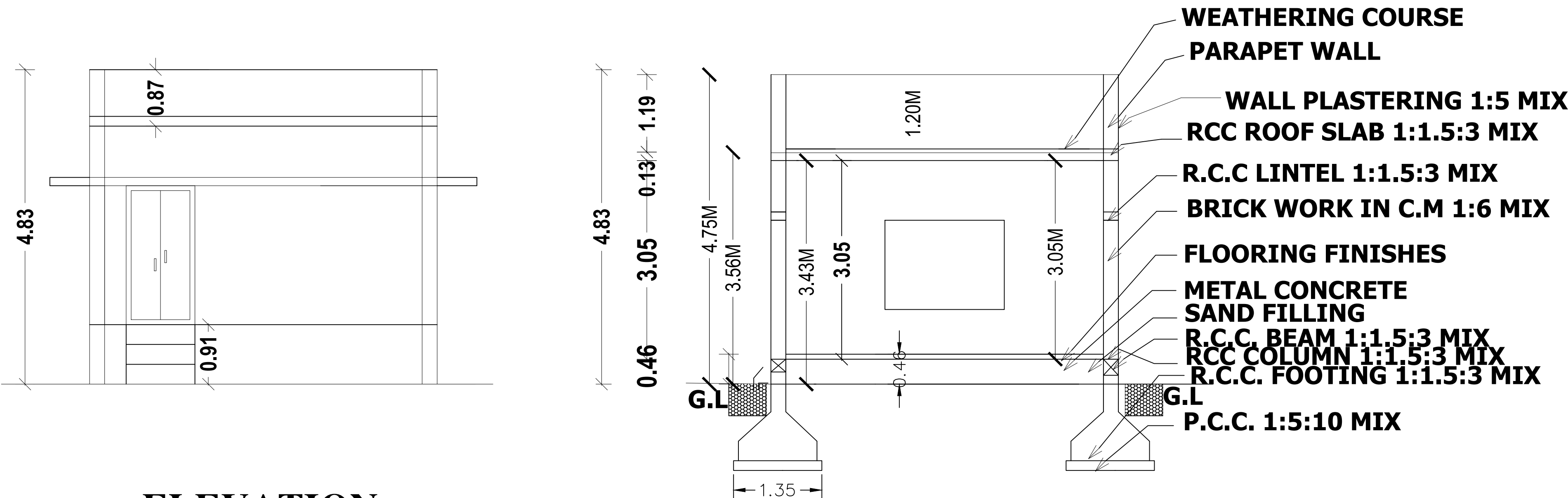
ELEVATION
