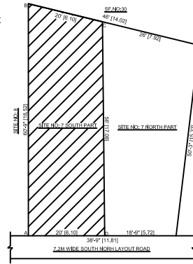
AREA OF THE SITE 'ABCD' SUBDIVISION PLAN
