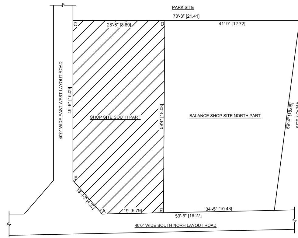
AREA OF THE SITE 'ABCDE' SUBDIVISION PLAN
