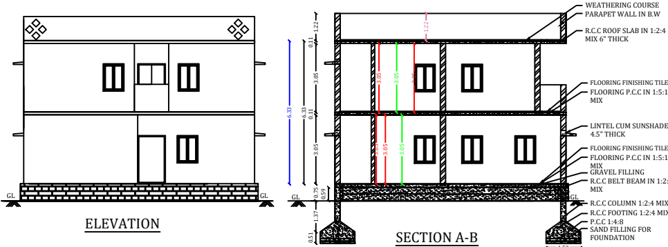
SECTION A-B
