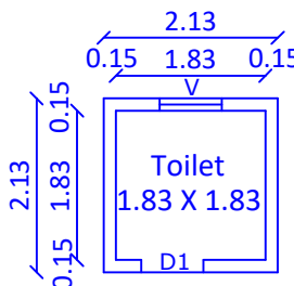
TOILET PLAN
