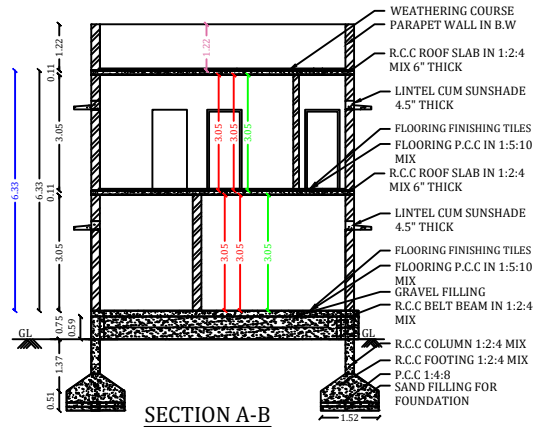
SECTION A-B
