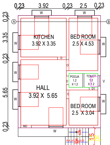
PRO. ADDI. FIRST FLOOR PLAN
