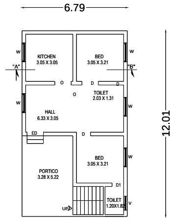
EXG.G.F.PLAN
