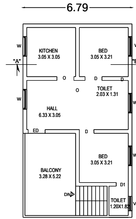
PRO.ADD.F.F.PLAN
