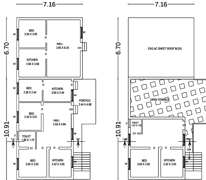
PRO.ADD.F.F.PLAN
