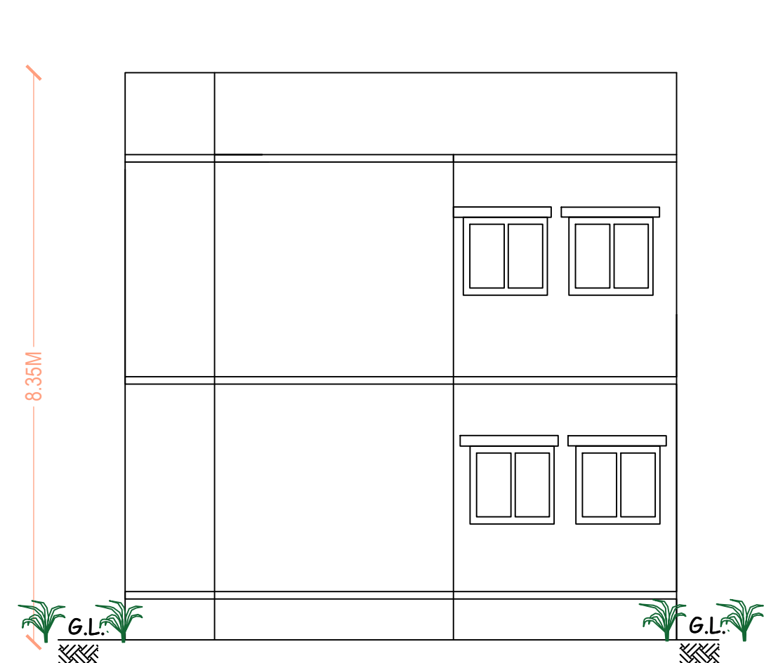
Elevation
