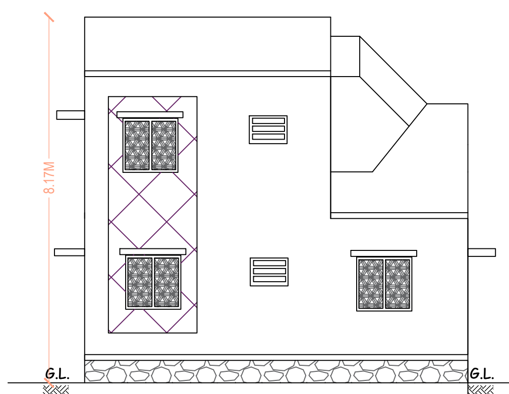
ELEVATION
