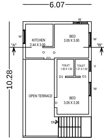
PRO. ADD. F.F PLAN
