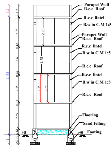
SECTION A-B
