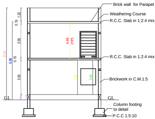
SECTION A-B
