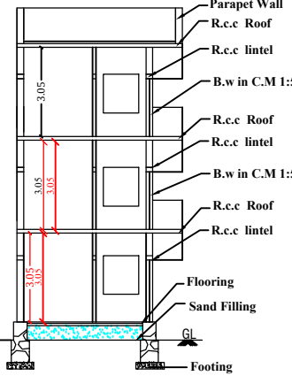
SECTION A-B
