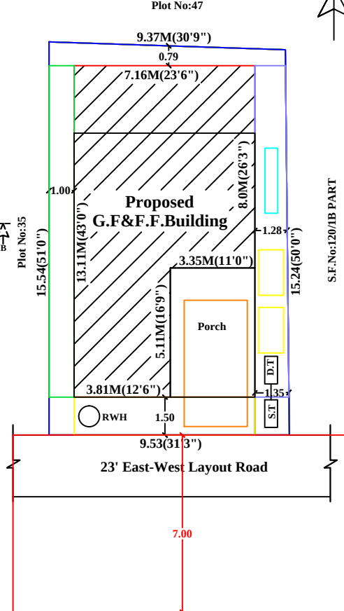
SitePlan
