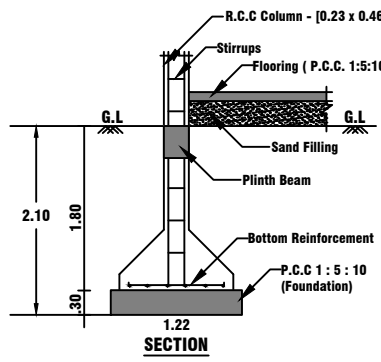
1:22 SECTION
