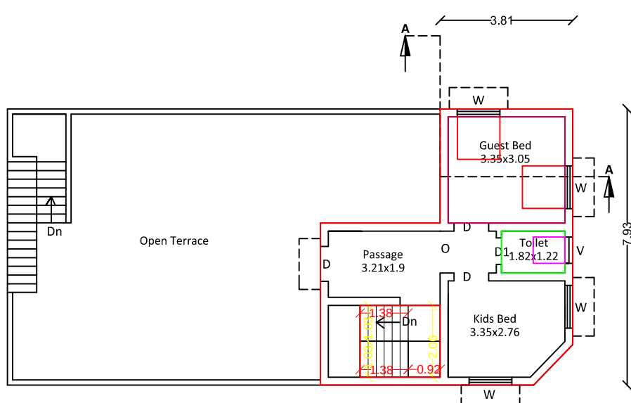
PRO FF PLAN
