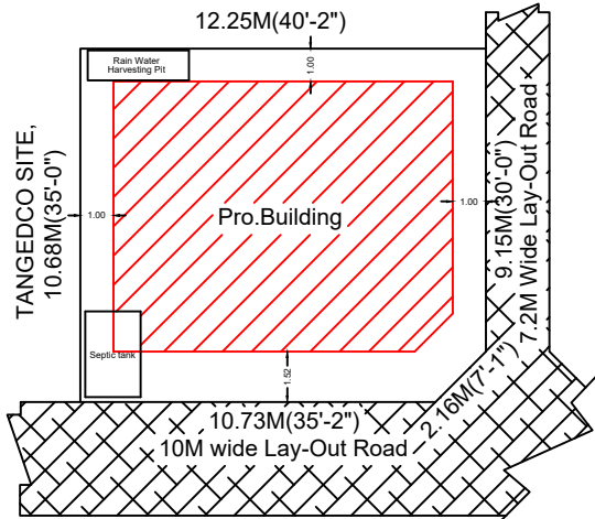
SITE PALN
