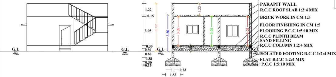
ELEVATION
