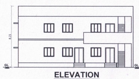
ELEVATION
