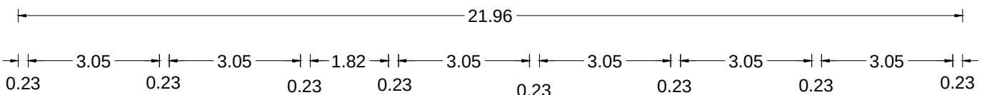
ELEVATION
