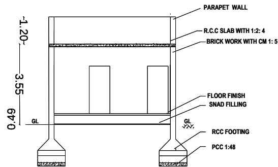
SECTION A-B
