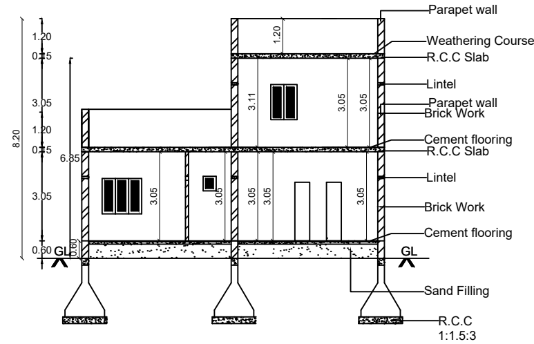
SECTION ON'AB'
