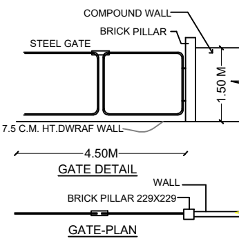
GATE-PLAN
