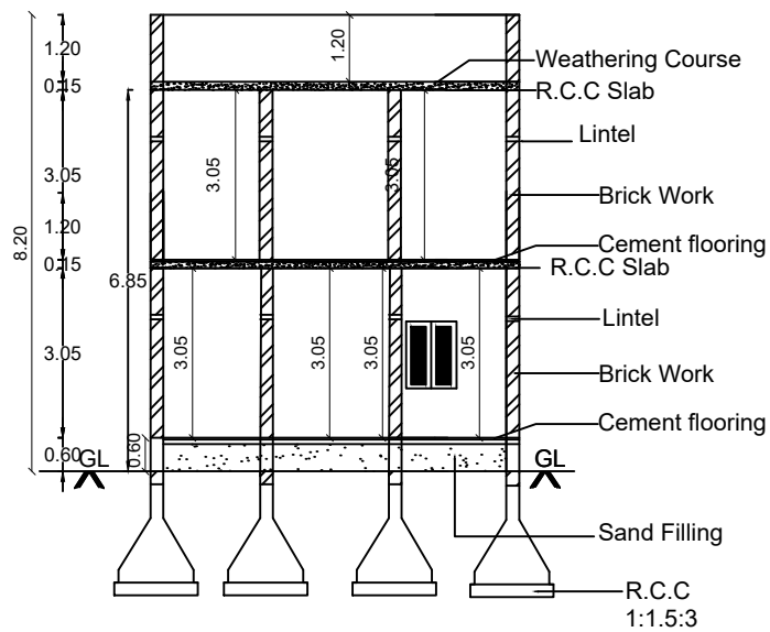
SECTION A-B
