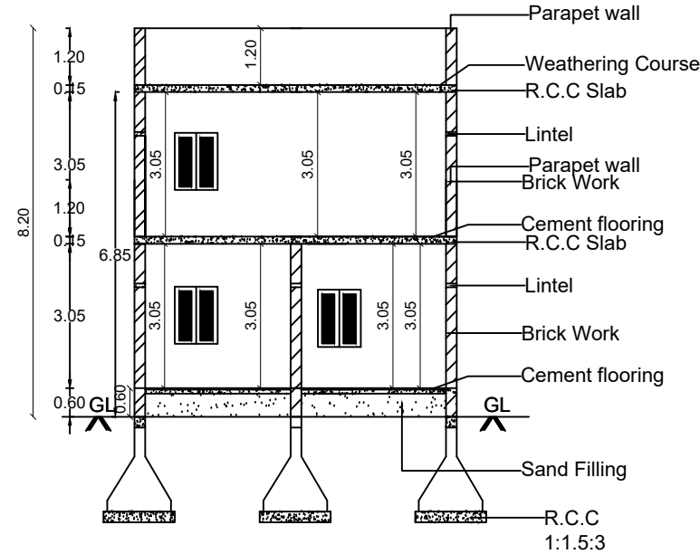
SECTION A-B
