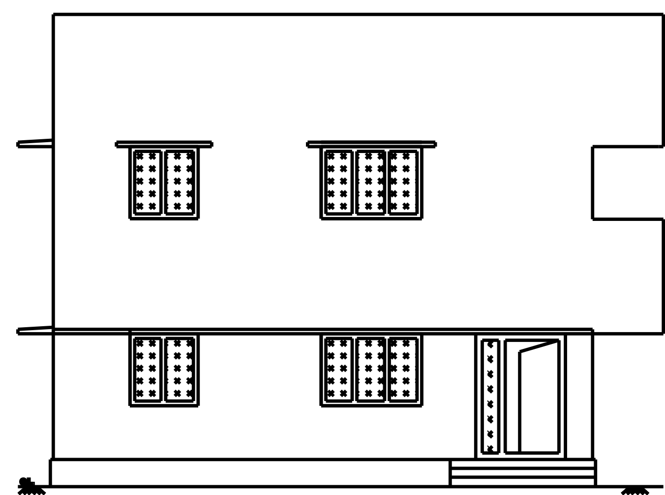
ELEVATION
