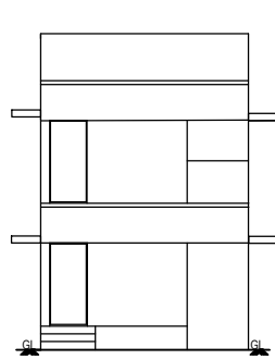
ELEVATION
