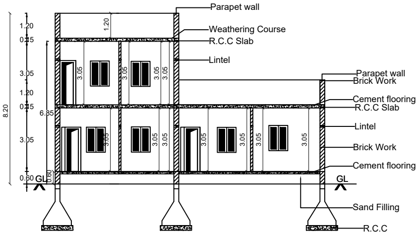
SECTION A-B
