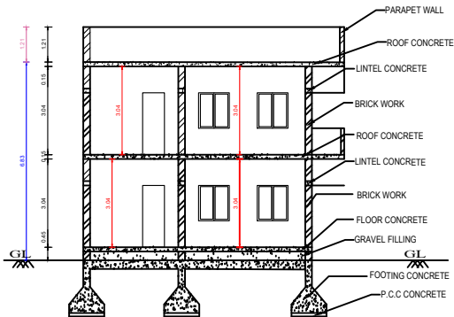
SECTION A-B
