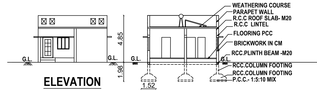
SECTION A-A
