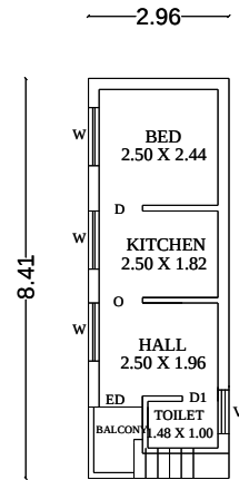
F.F. PLAN
