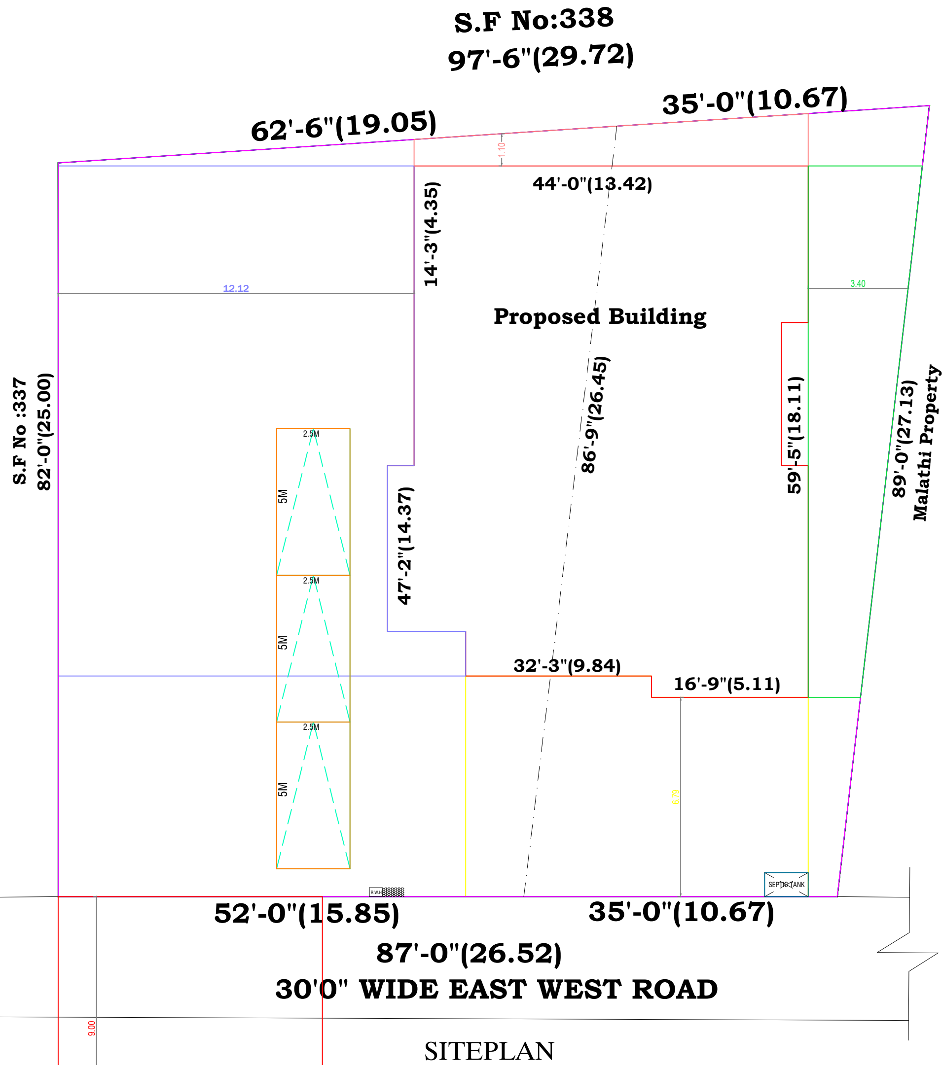
SITEPLAN
