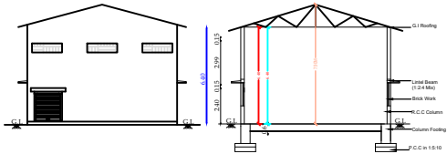
Elevation
