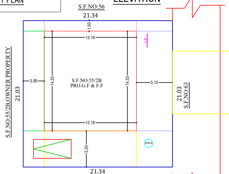
S.F.NO:55/2B,OWNER PROPERTY
