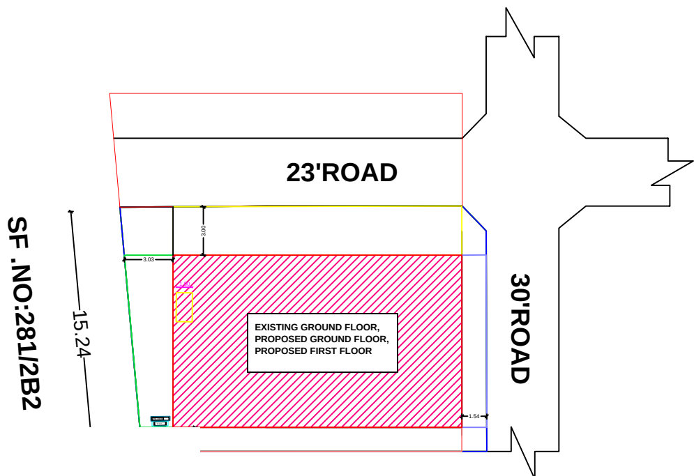
SITE NO:33 SITE PLAN
