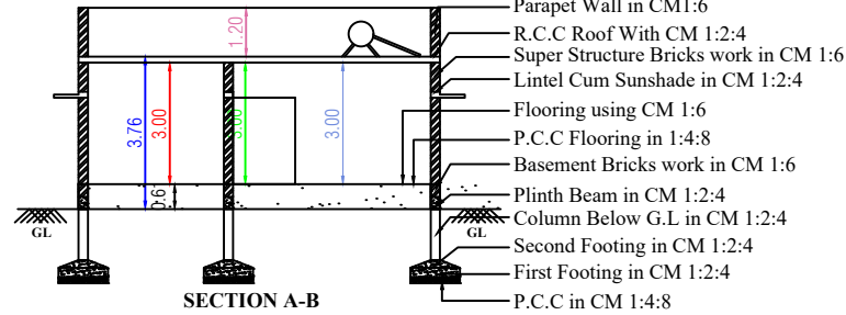
SECTION A-B
