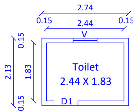
TOILET PLAN
