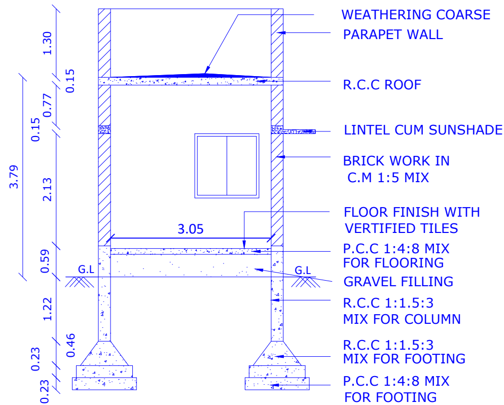
SECTION A-A'
