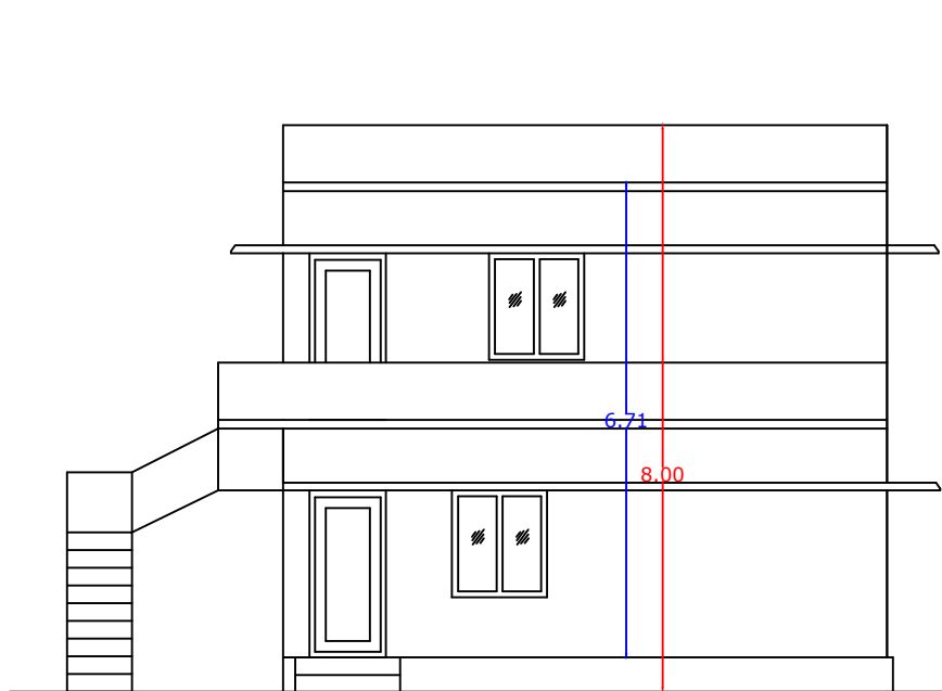
ELEVATION
