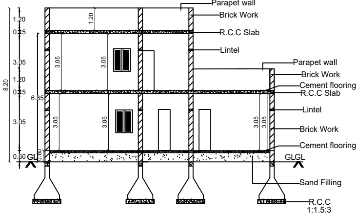
SECTION A-B
