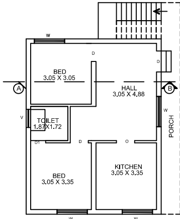
PRO.. G.F PLAN
