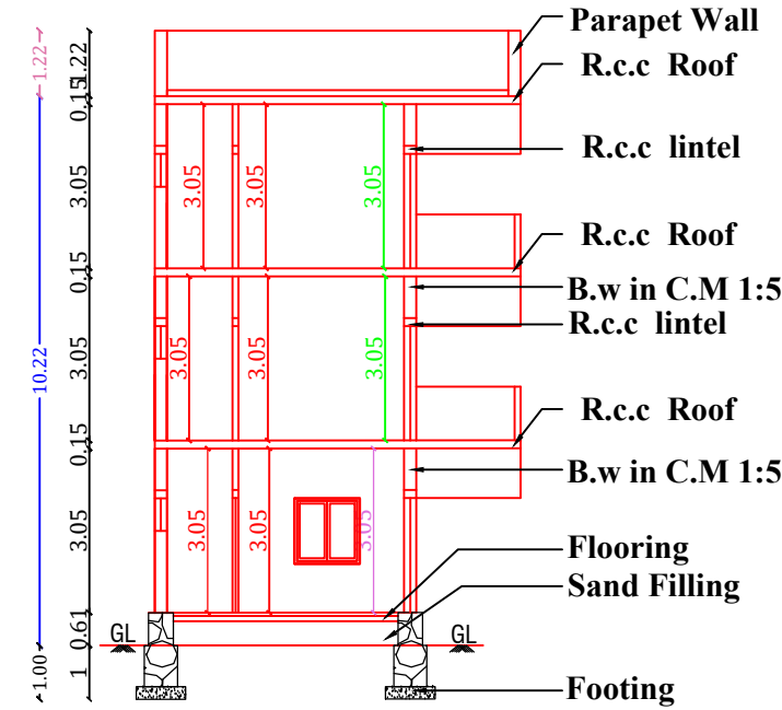
SECTION A-B
