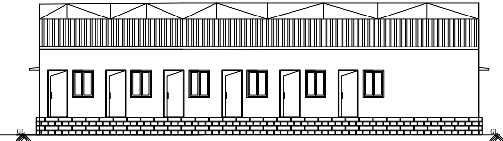
ELEVATION
