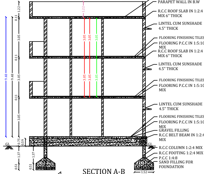
SECTION A-B
