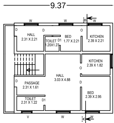
PRO. ADD. F,F PLAN
