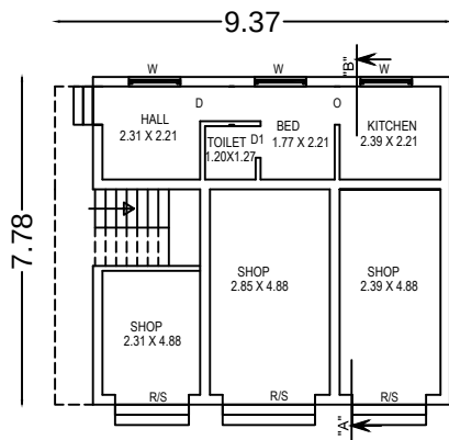
EXG. G.F. PLAN
