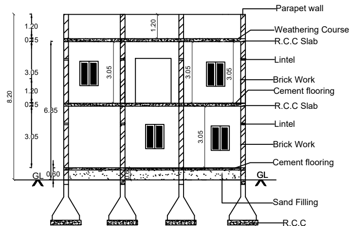
SECTION A-B
