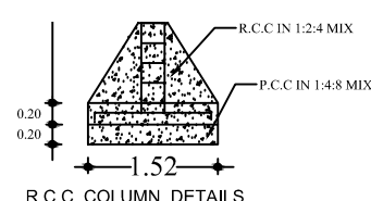
R.C.C. COLUMN
