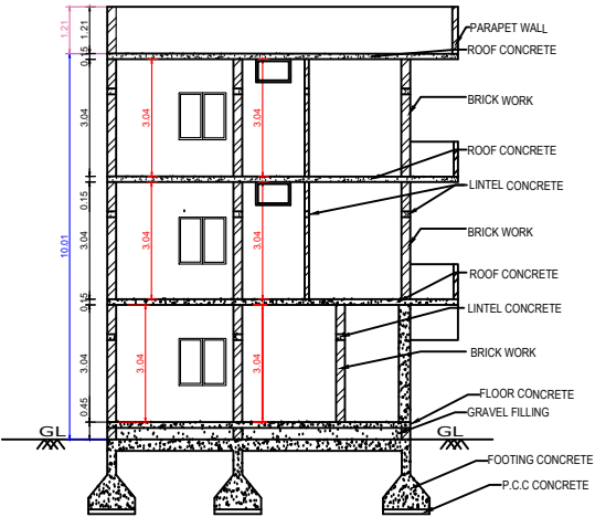
SECTION A-B
